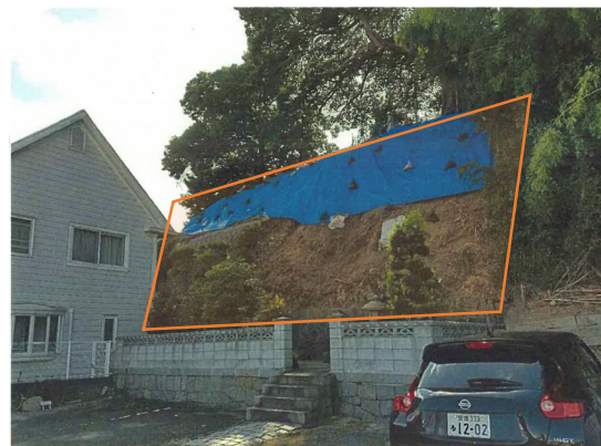
急傾斜地法面对策：施工前
