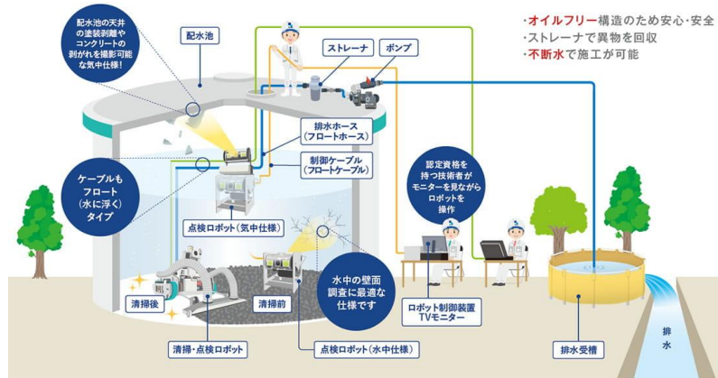
図表 2 ロボットを用いた施工概要
